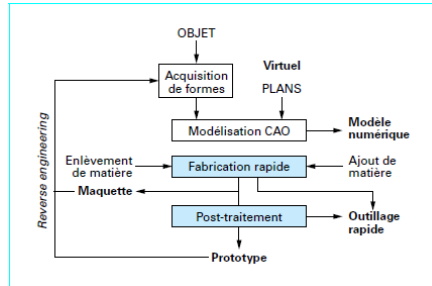
Processus de prototypage rapide (T1 BM7 017)
